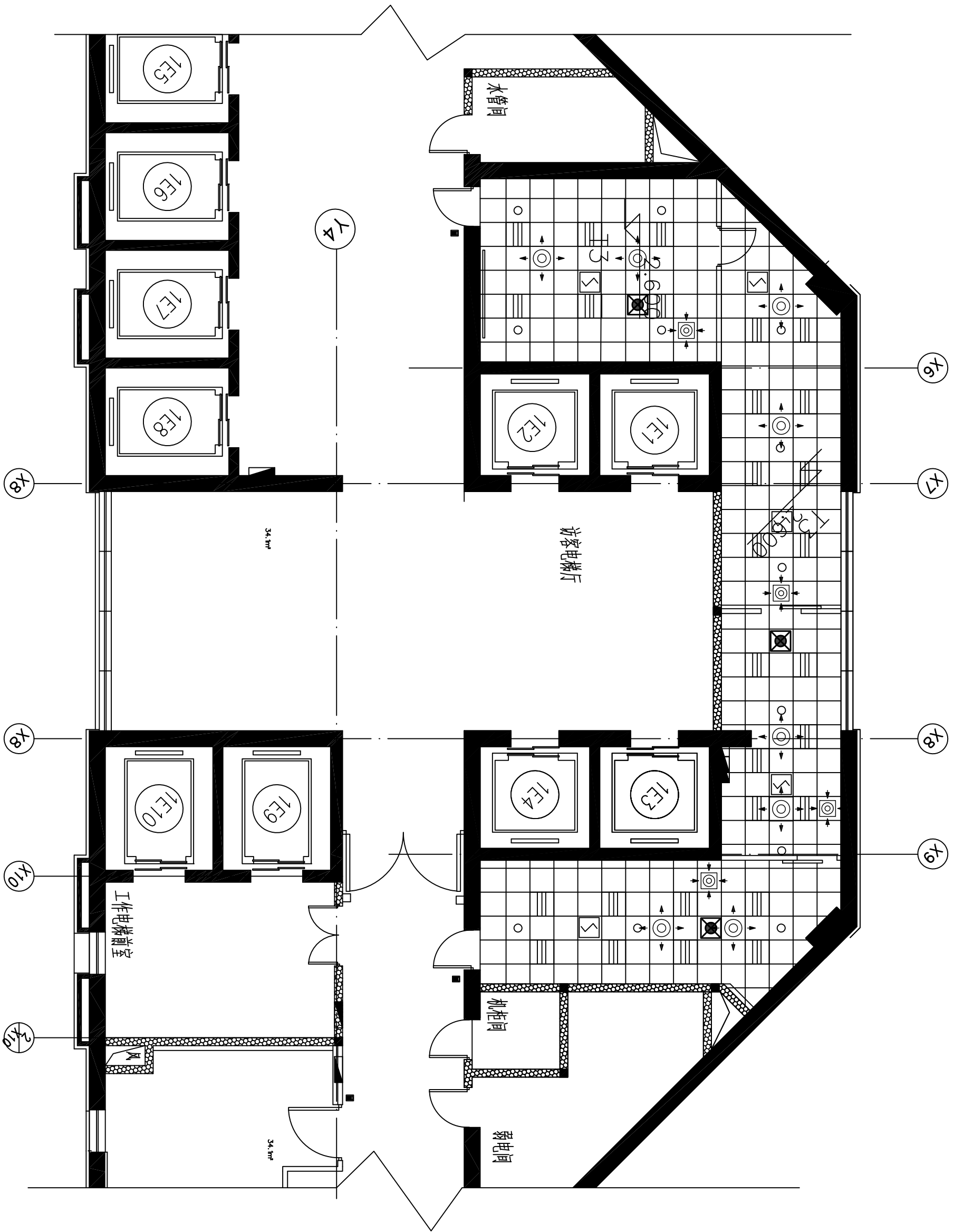
10F神经中心天花排布图 1:100
