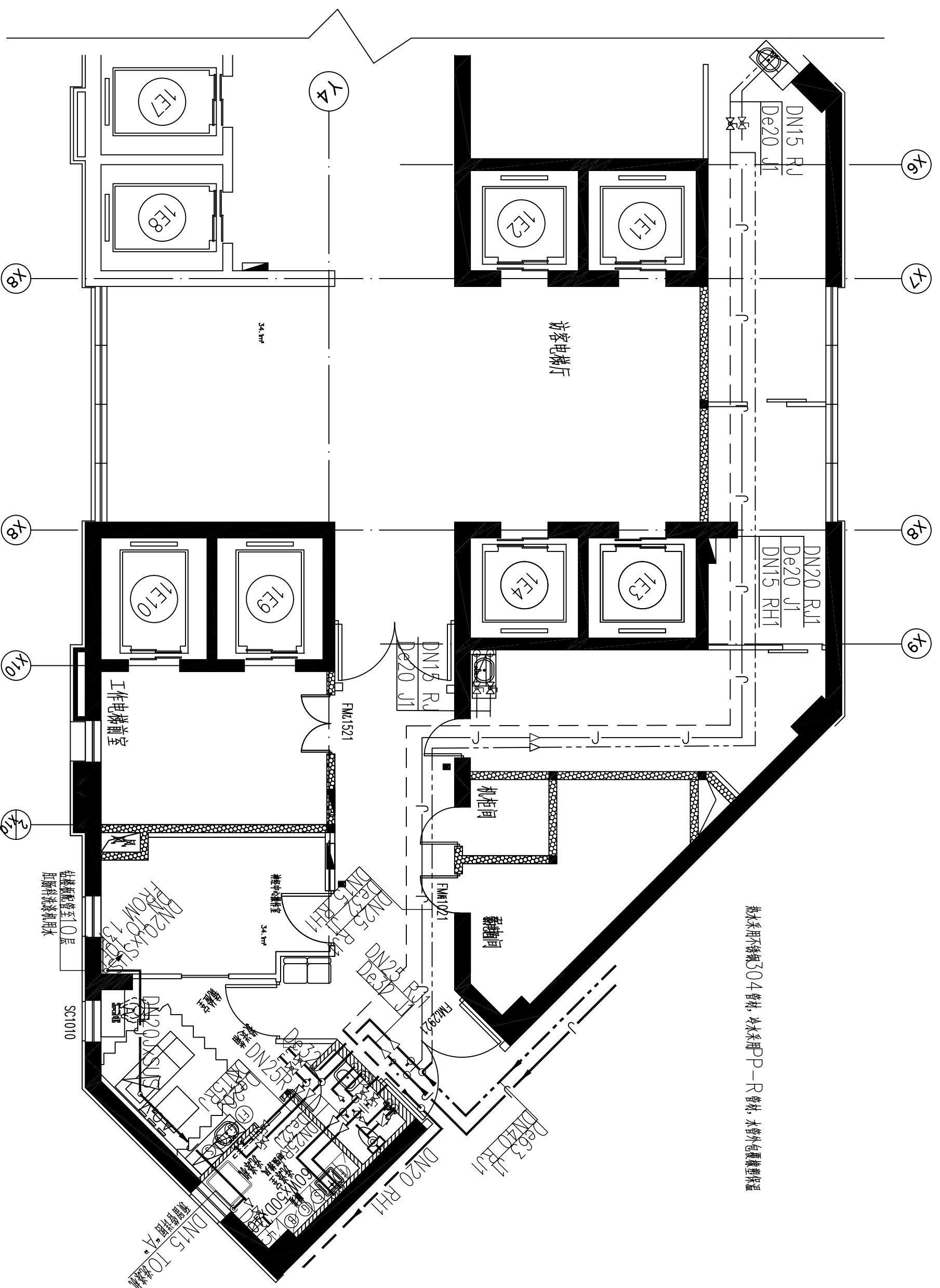
10F神经中心给水平面图 1:100
