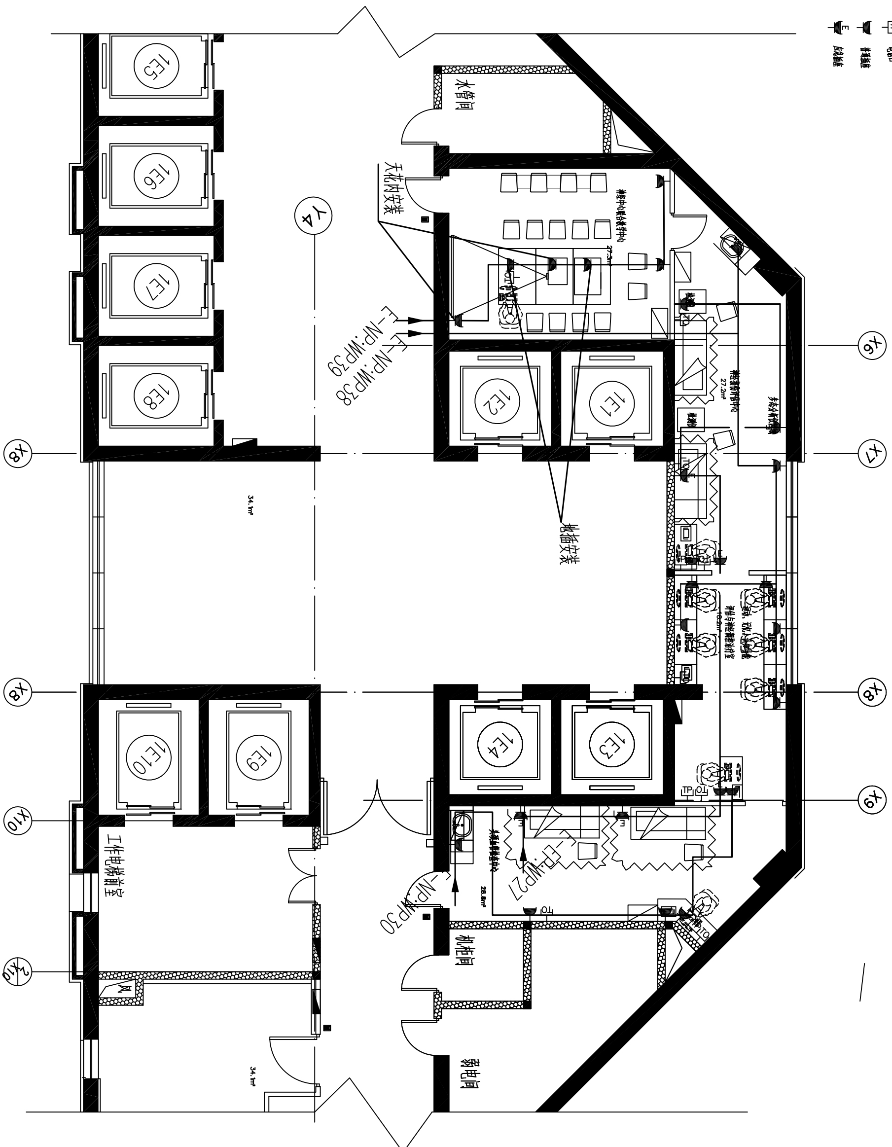
10F神经内科中心插座平面图 1:100
