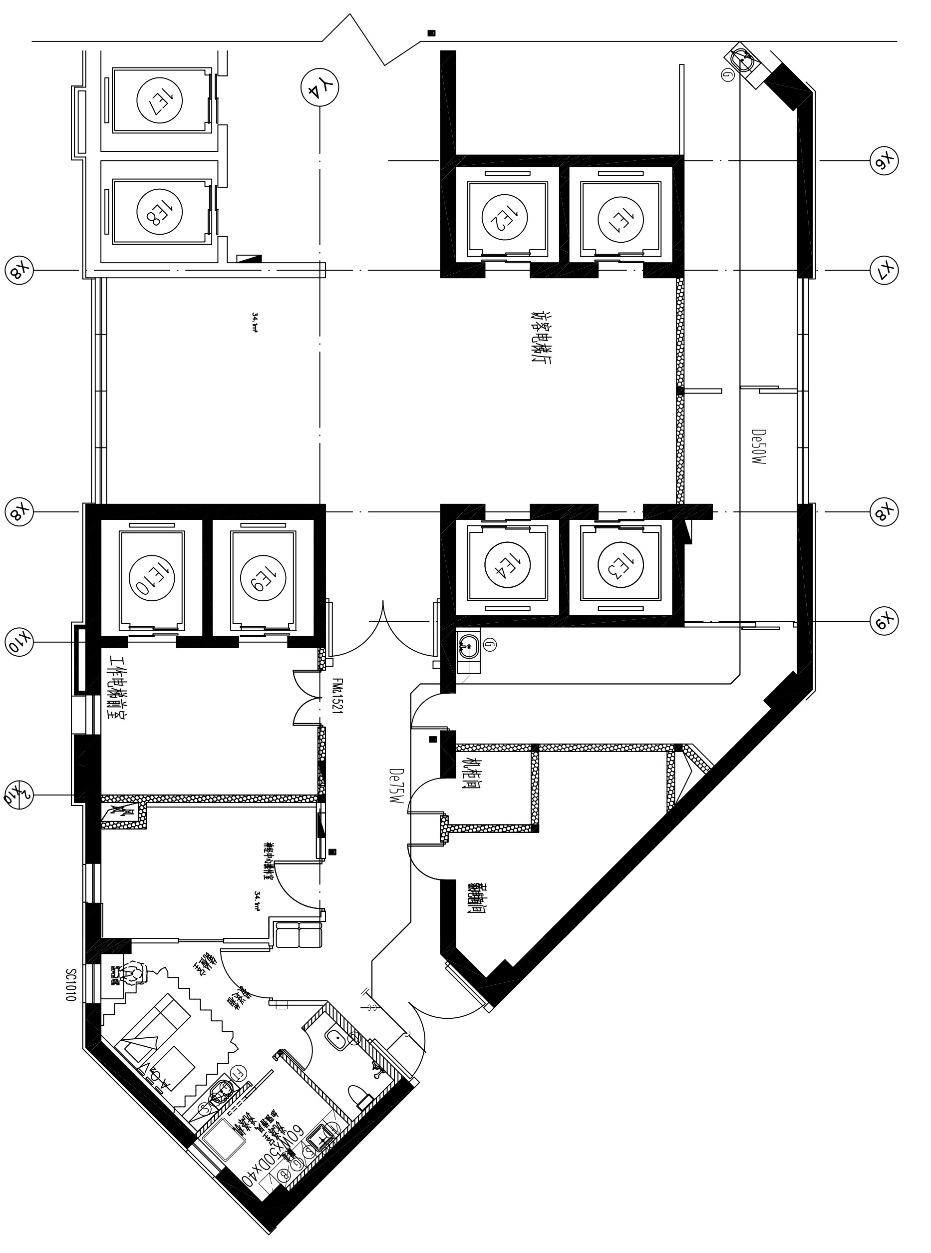
10F神经中心排水平面图 1:100
