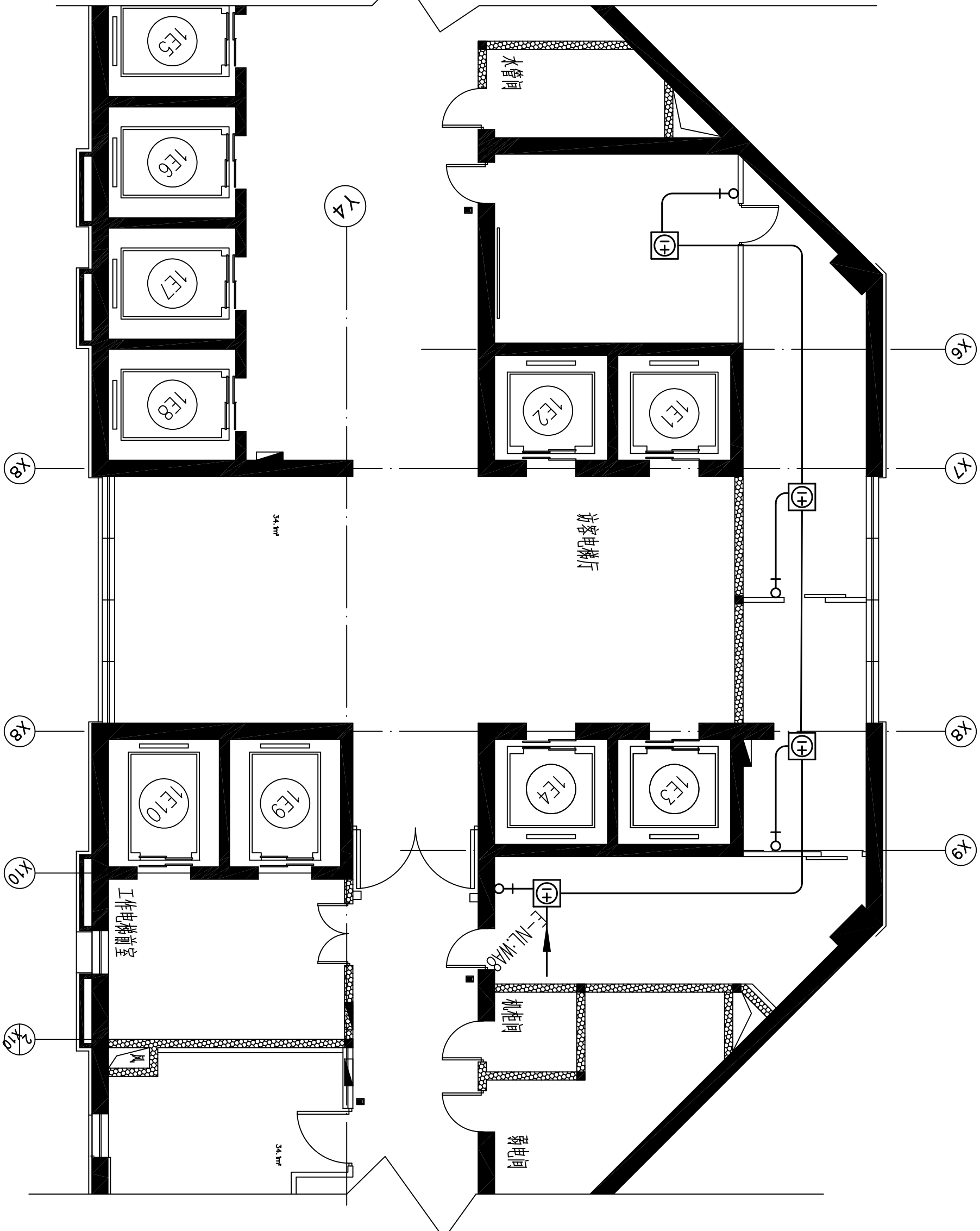
10F神经中心空调电气图 1:100
