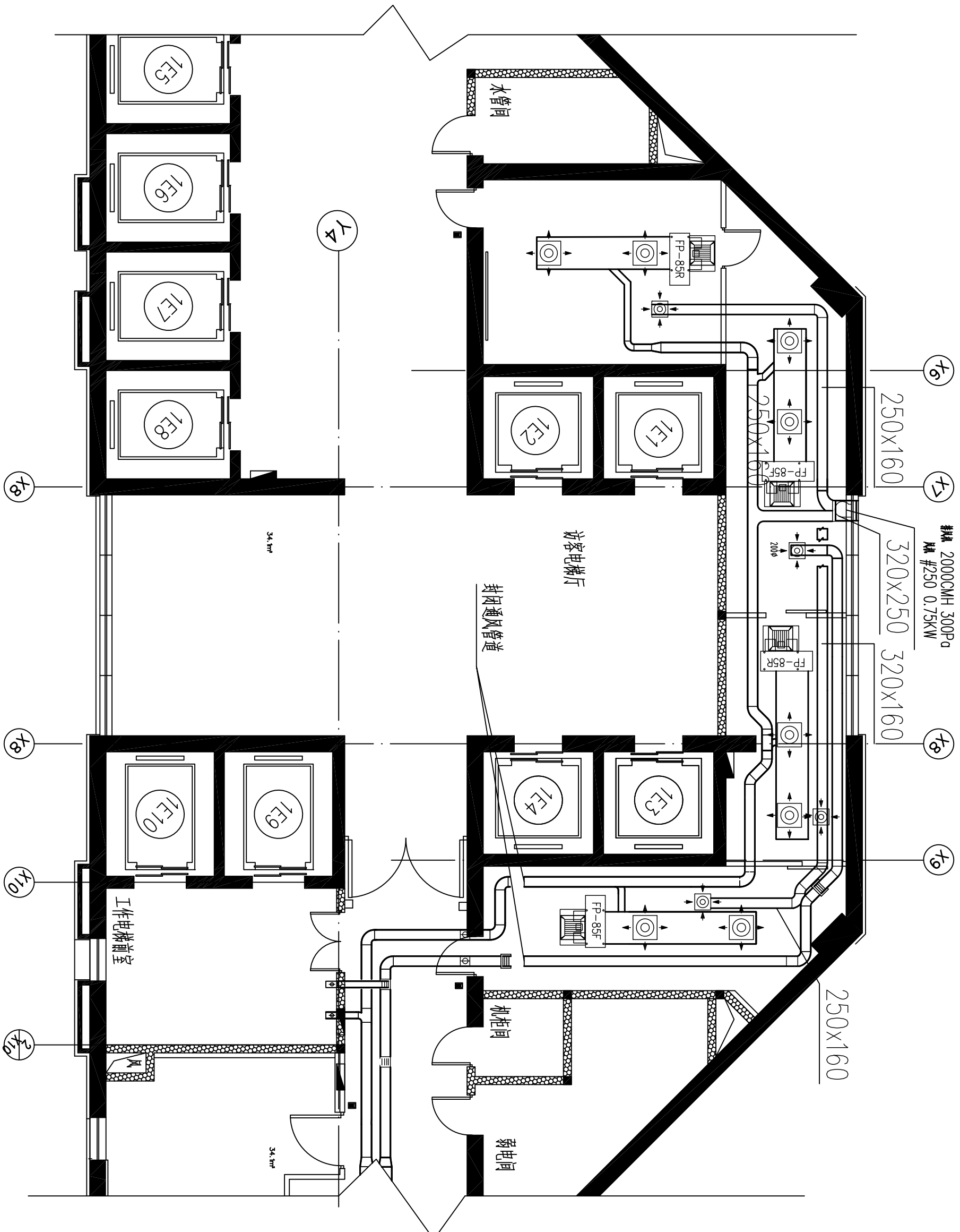
10F神经中心空调风管图 1:100
