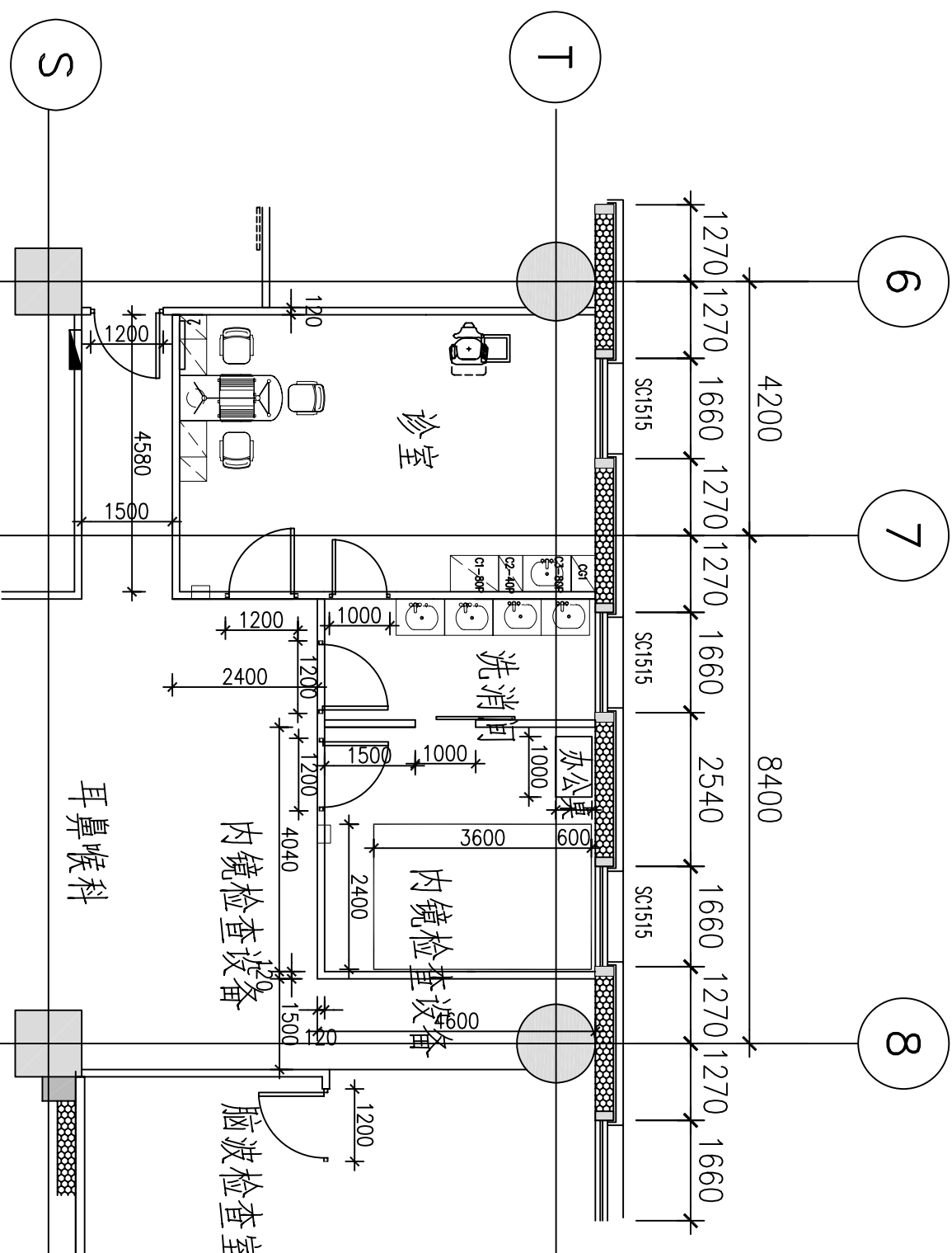
新洗消间和内镜检查室（平面图）
